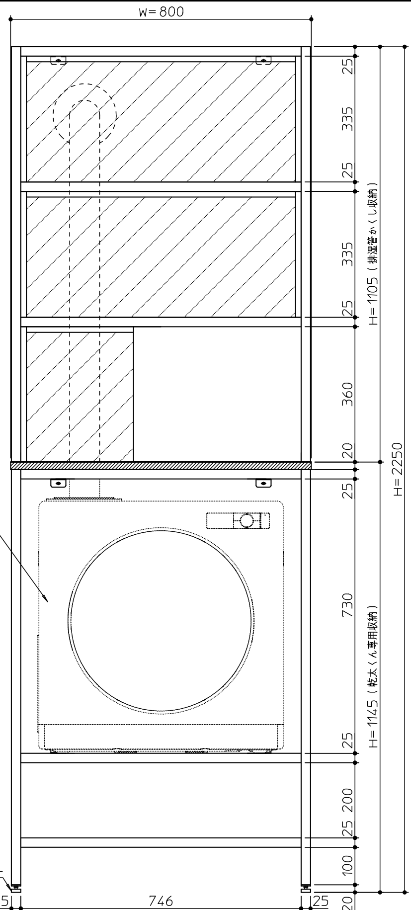
正面図
