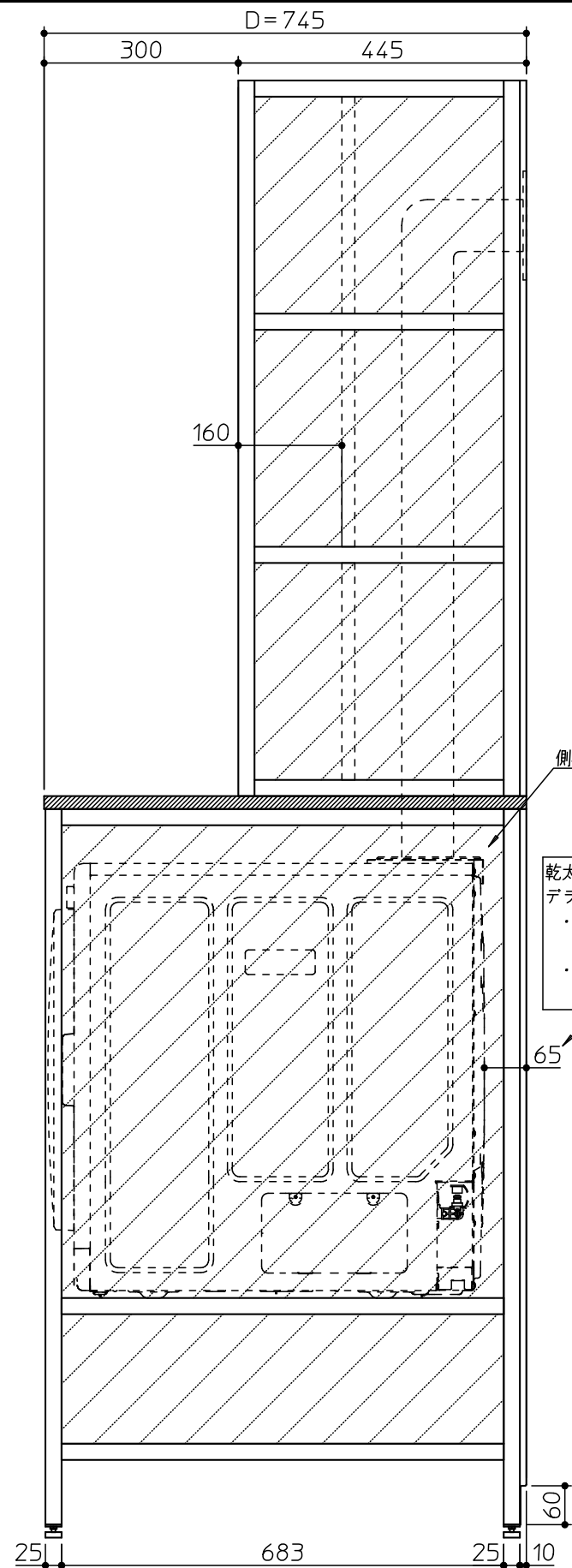
側面図
