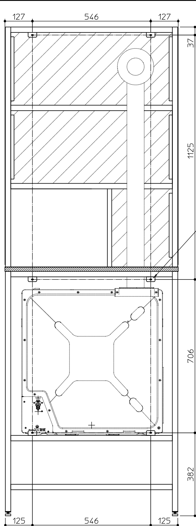
背面図
