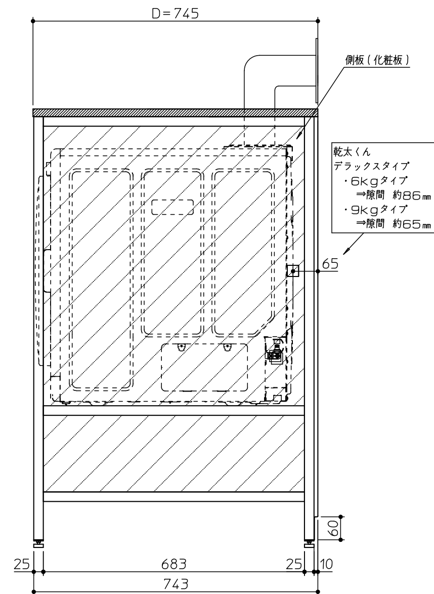
側面図
