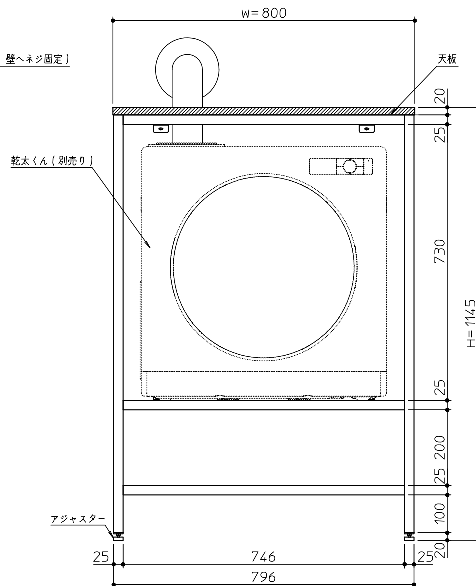
正面図
