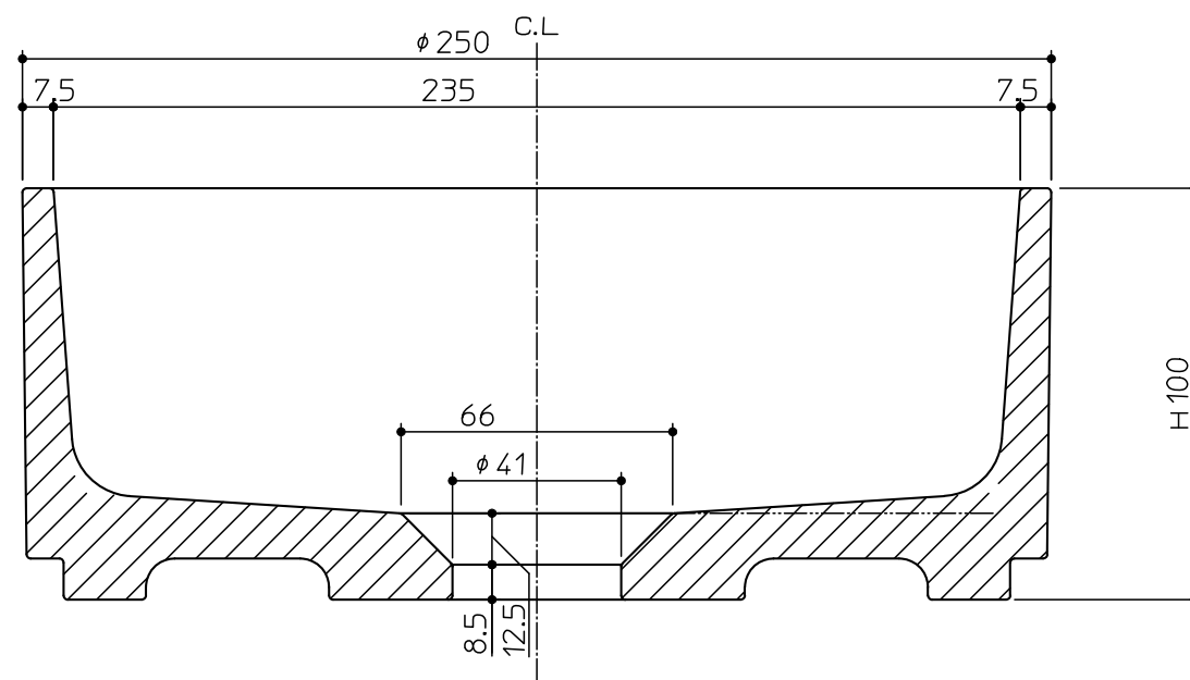
A-A' 断面
