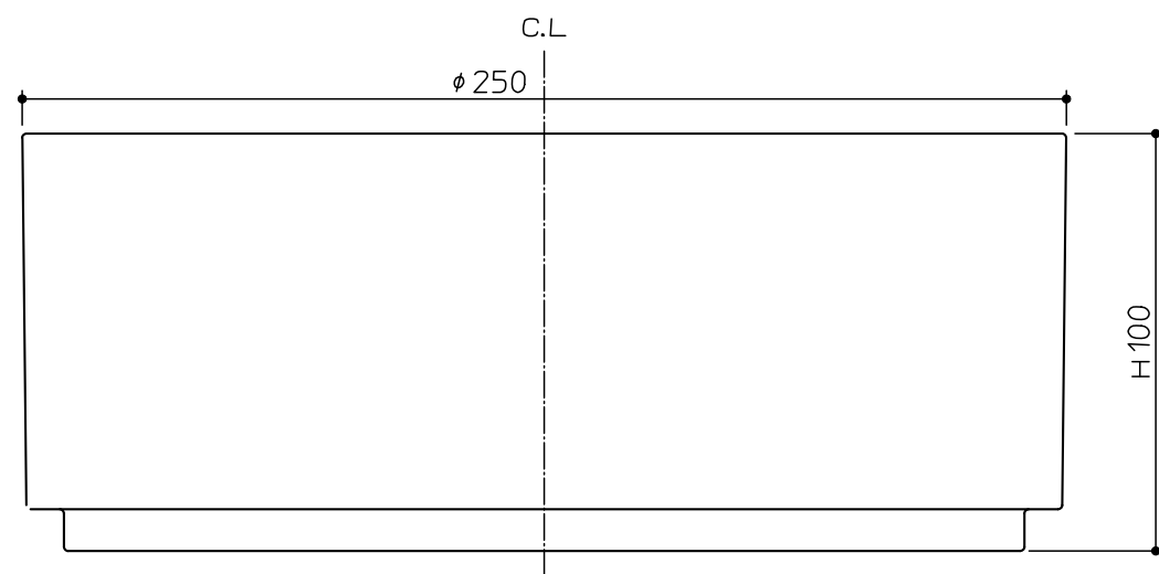
正面図
