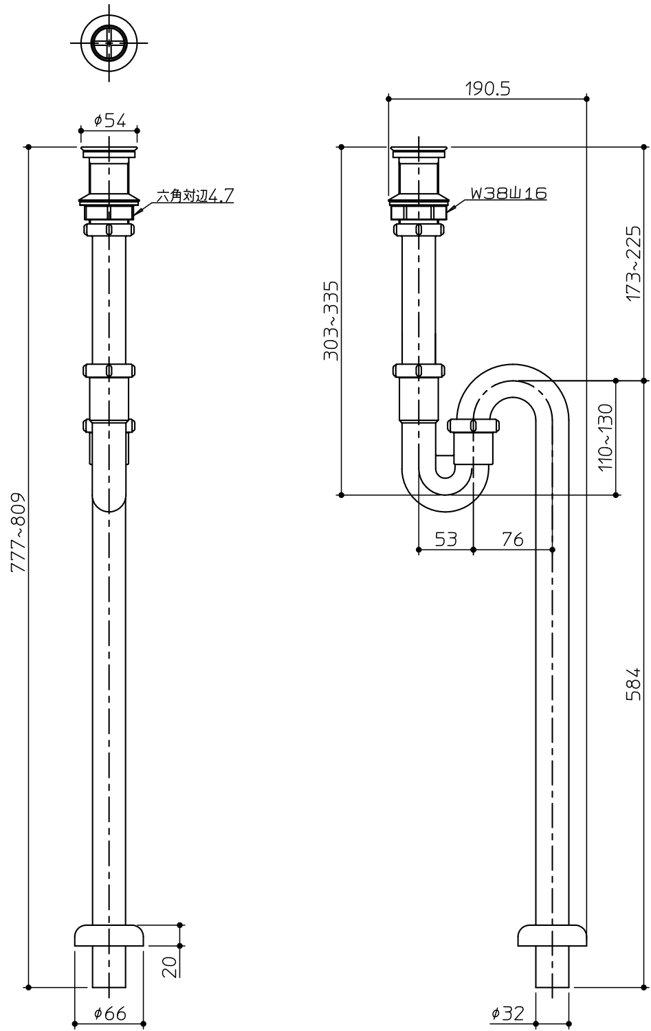
排水口内部形状
